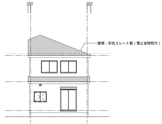
北立面図 S=1:100
