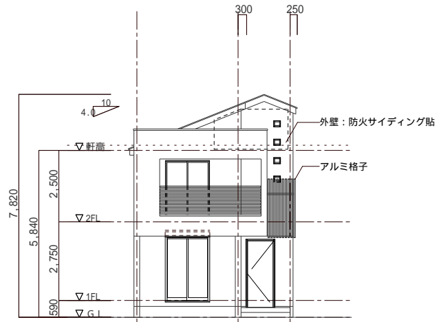
南立面図 S=1:100
