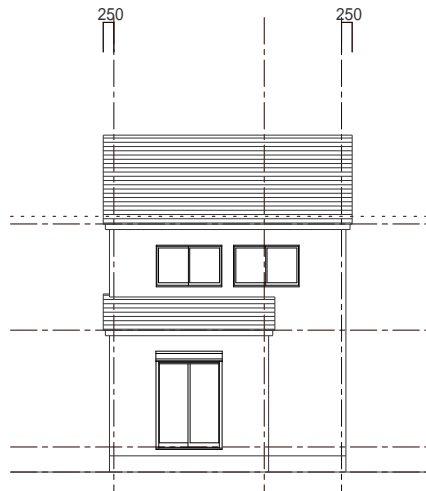
北立面図 S=1:100
