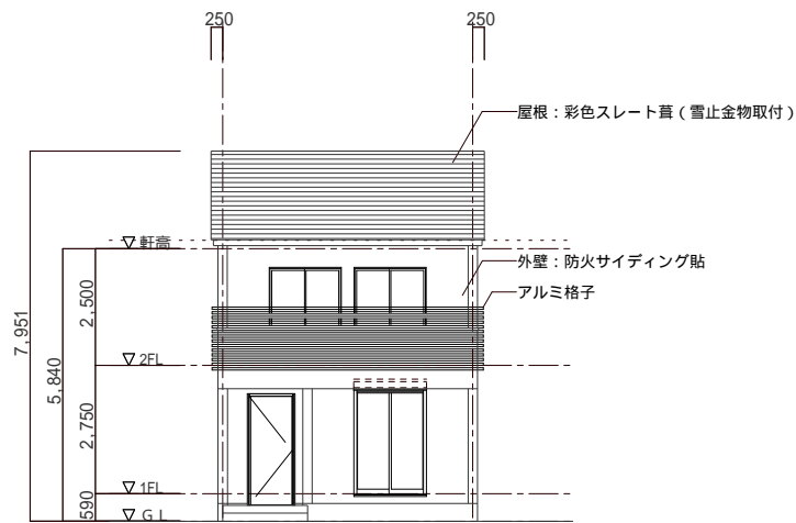
南立面図 S=1:100
