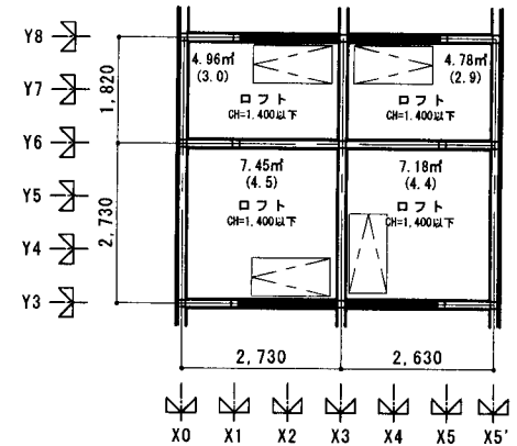
ロフト平面図 S=1:100
